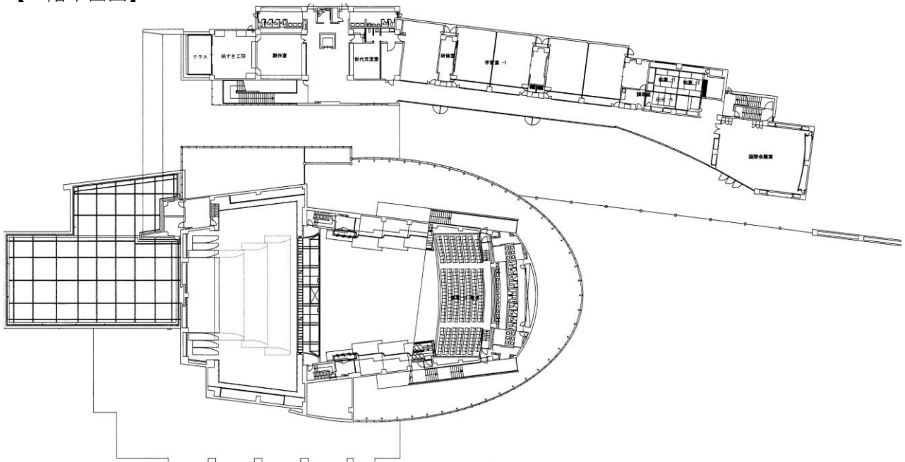
【三階平面図】
