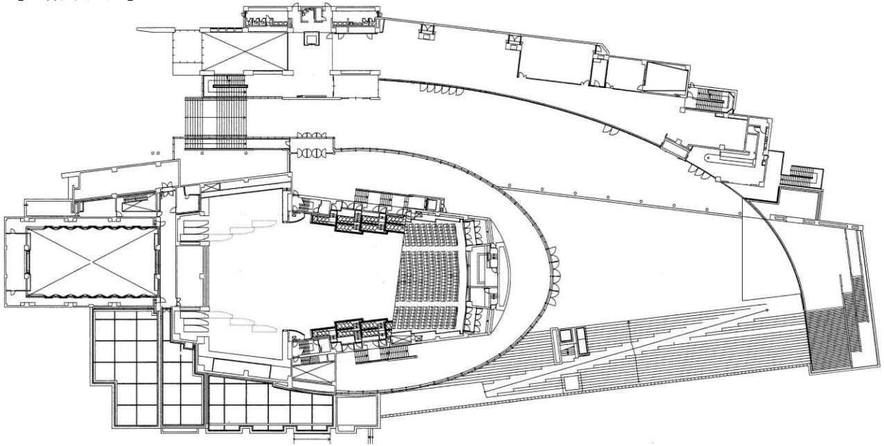
【二階平面図】
